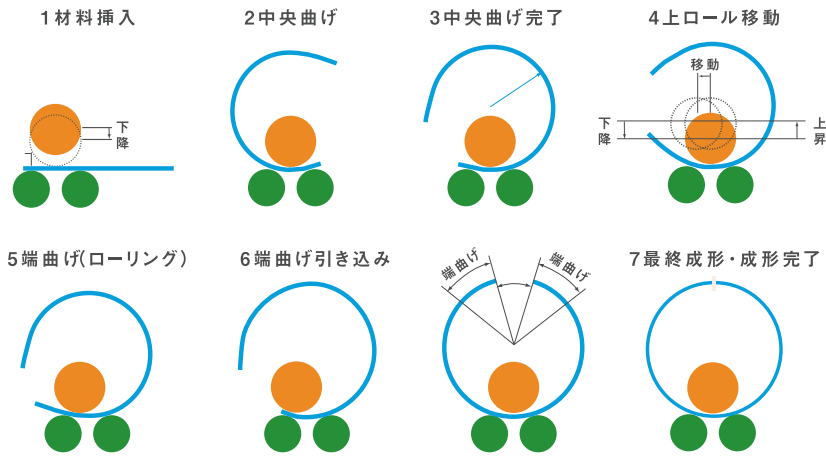
SR-DH(手動加圧式、端曲げ機能付)仕様
